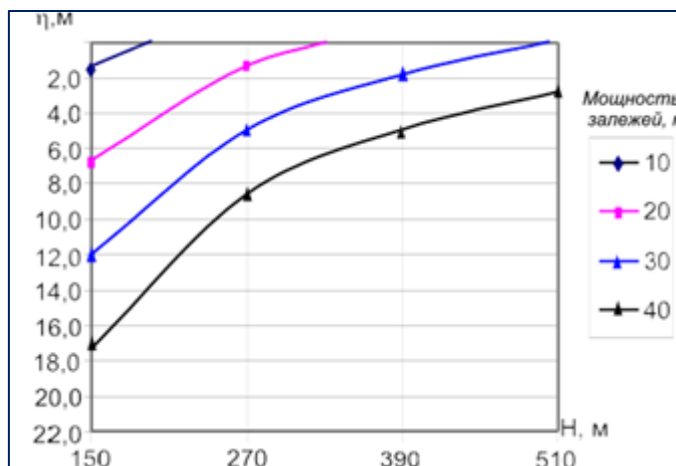
Рисунок 1 – График зависимости величины оседания земной поверхности от мощности m , глубины разработки H при K_p=1,03 при разработке пологих залежей из однотипных горных пород
