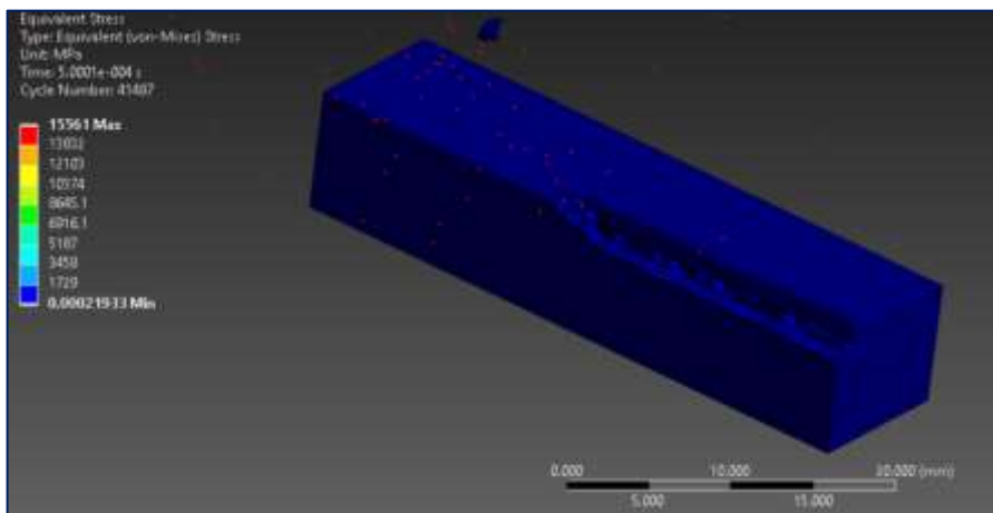
Рисунок 2 – Эквивалентное напряжение в заготовке
