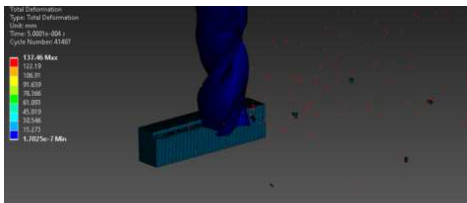
Рисунок 4 – Стружкообразование при фрезеровании концевой фрезой
