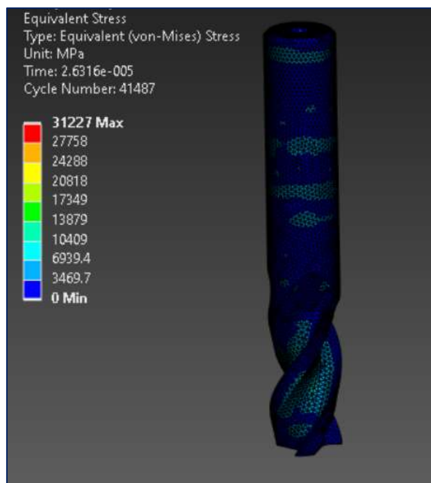
Рисунок 3 – Эквивалентное напряжение в концевой фрезе
